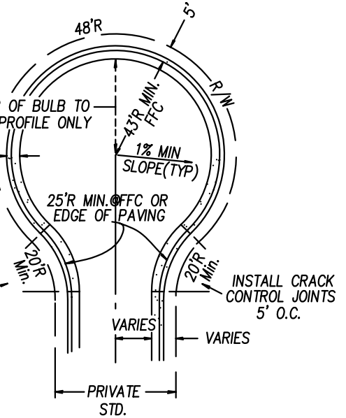
PAVED PERMANENT N.T.S.
