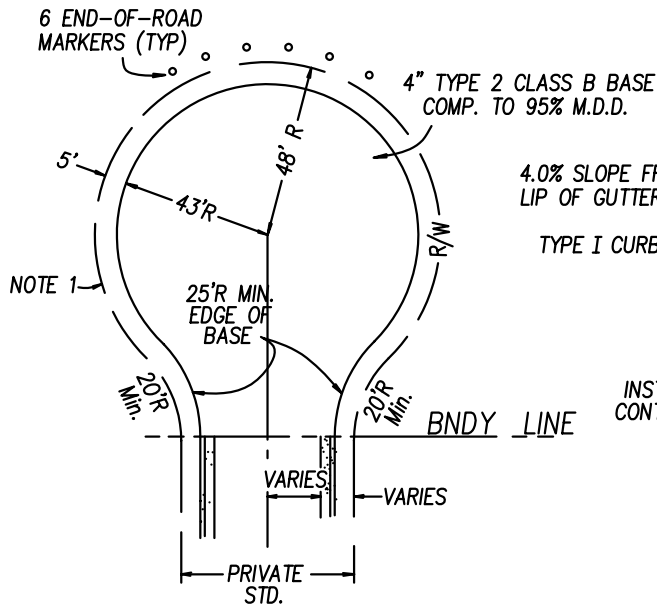
UNPAVED TEMPORARY N.T.S.
