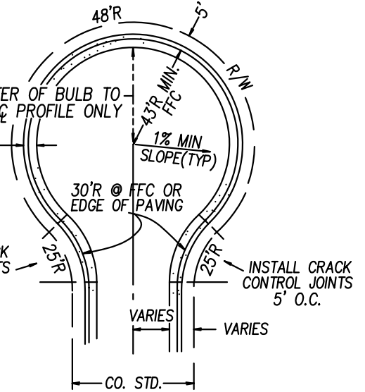
PAVED PERMANENT N.T.S.
