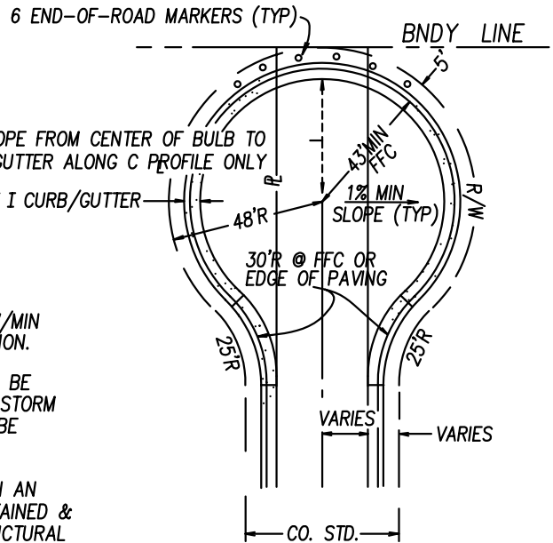
PAVED TEMPORARY N.T.S.
