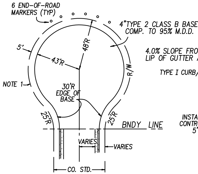
UNPAVED TEMPORARY N.T.S.
