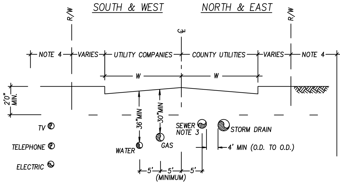
TYP. SEC. N.T.S.
